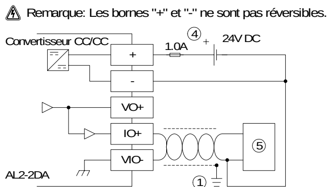
Figure 11.4: Câblage pour la sortie d'un courant
