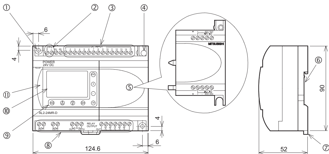
Abbildung 1.2: Bedienungselemente(AL2-14MR-*,AL2-24MR-*)
