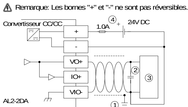
Figure 11.3: Câblage pour la sortie d'une tension
