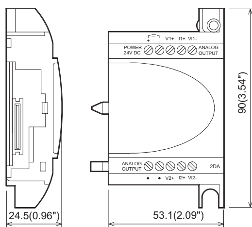
Figura 11.1: Dimensiones exteriores
