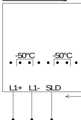
Figur 13.5: Avstämning av offset för AL2-2TC-ADP
