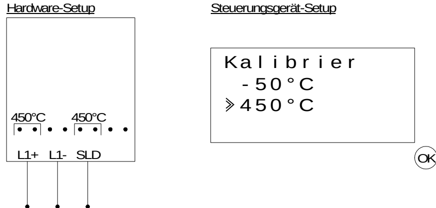
Abbildung 13.7: Abgleich der Verstärkung beim AL2-2TC-ADP
