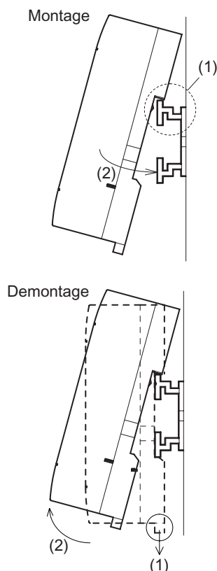
Abbildung 12.3: Installation
