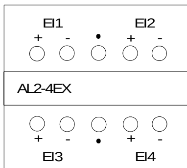
Figur 5.8: AL2-4EX-A2, likströmsingång
