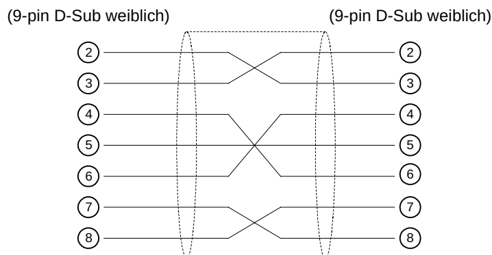
Abbildung 8.3: RS-232C seriellles Kabel Pin-Belegung
