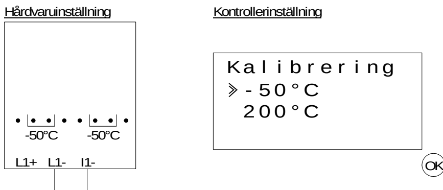
Figur 12.5: Avstämning av offset för AL2-2PT-ADP
