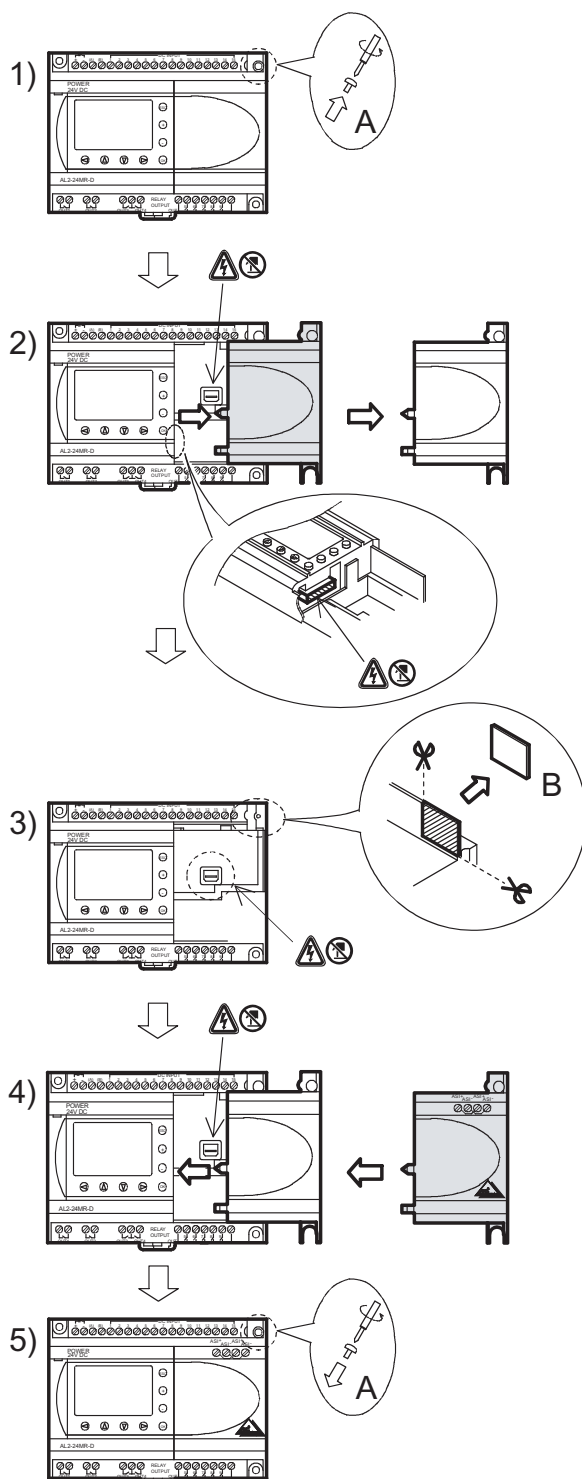
Figura 9.3: Instalación
