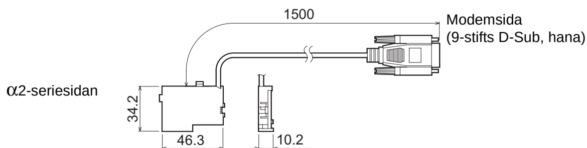
Figur 8.1: Yttre mått
