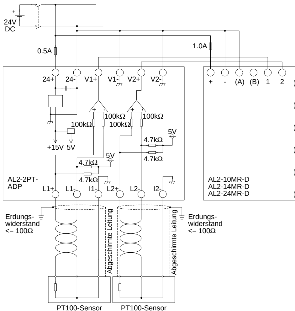
Abbildung 12.4: Anschluss
