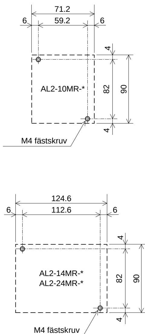
Figur 3.4: Direktmontering
