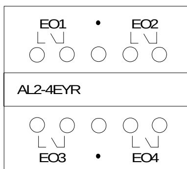
Figur 5.9: AL2-4EYR, reläutgång
