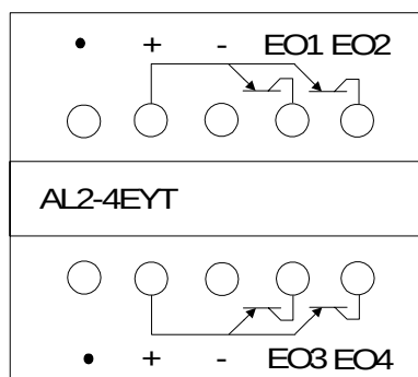
Abbildung 5.10: AL2-4EYT, Transistor-Ausgang
